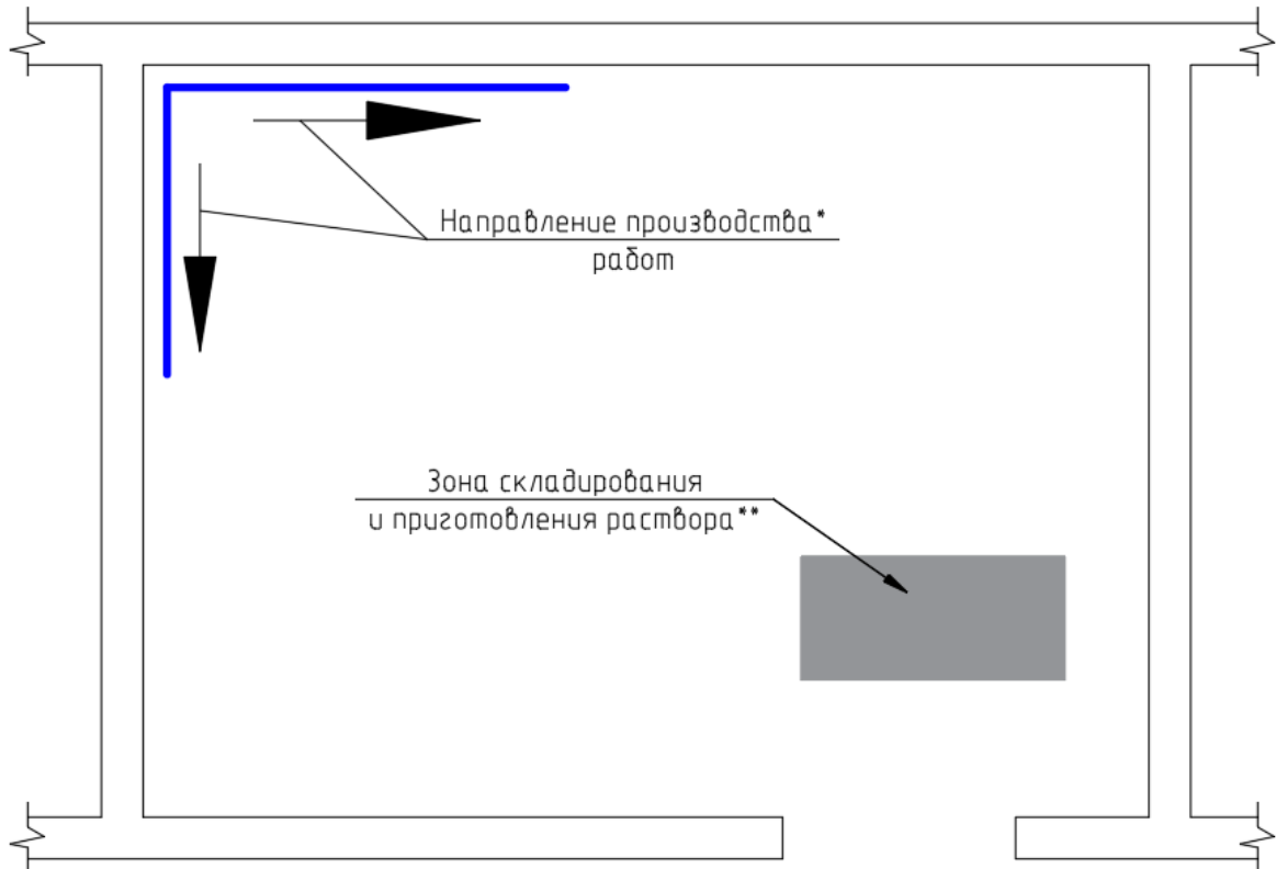
Рис.11. Схема организации работ (внутренние стены)
