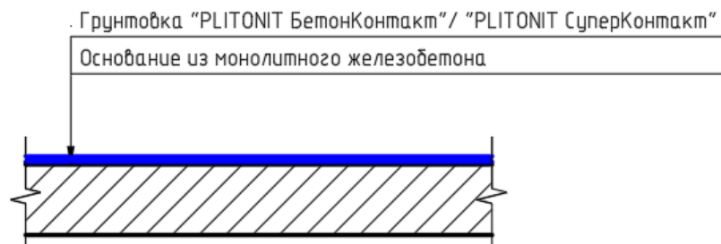
Рис.8. Конструктивный разрез №1.
