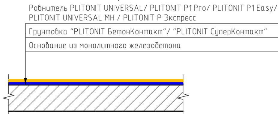
Рис.9. Конструктивный разрез №2.
